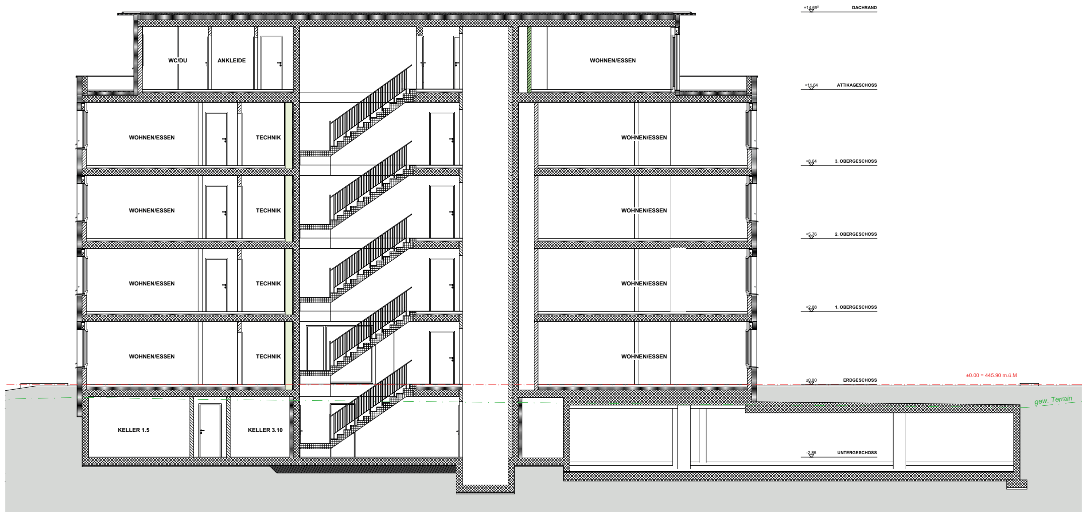
Schnitt B-B
